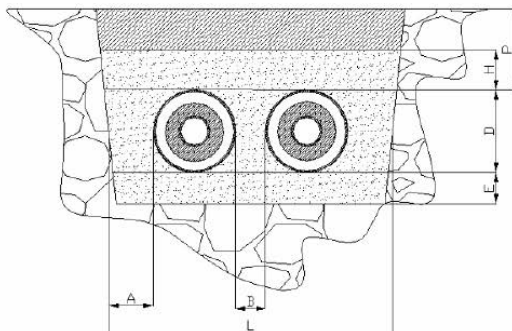
Schémas des tranchées Tucal – 1 tube / 1gaine et 2 tubes / 1 gaine
