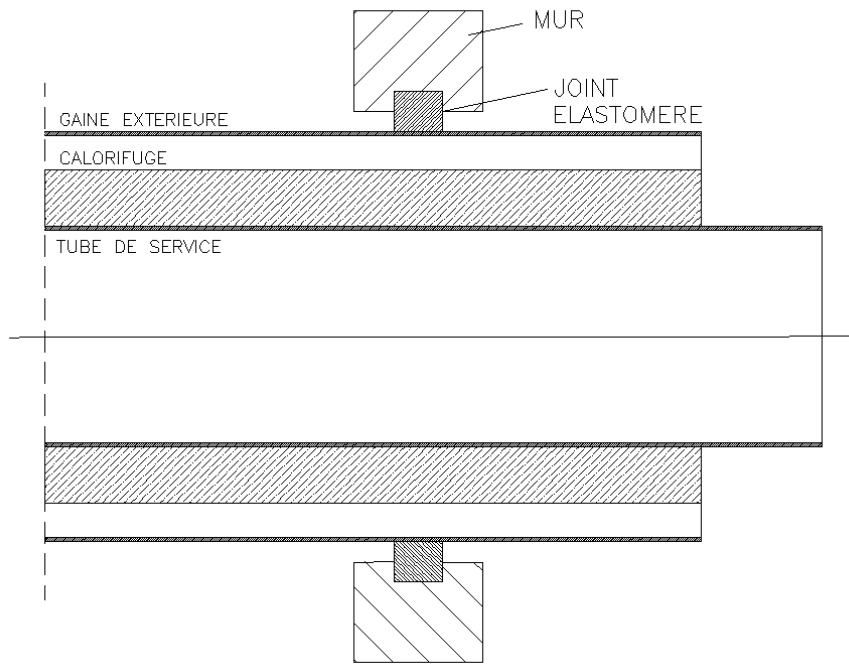
Figure 7 - Passage de cloison : joint élastomère
